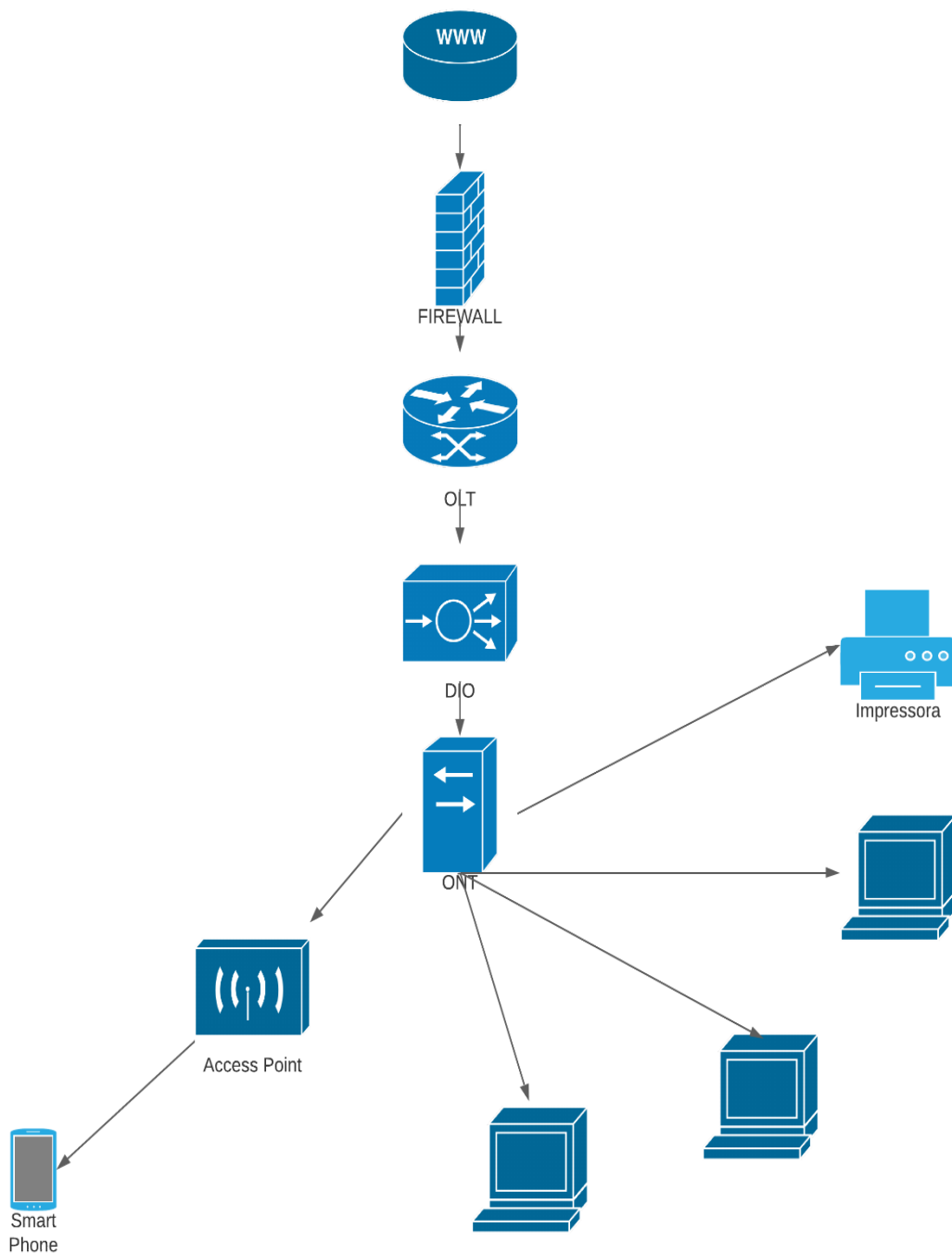
Figura 01 - Topologia da Rede Lógica
